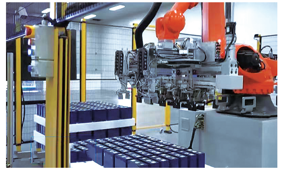
新疆首条储能锂电池生产线。 通讯员 米立克·哈力汗 摄
